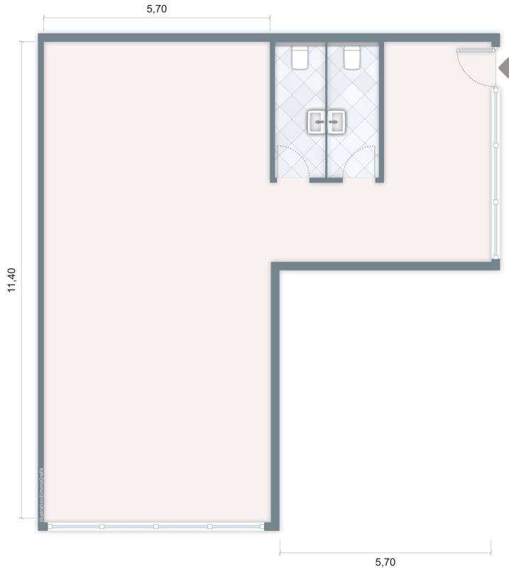
Grundriss
