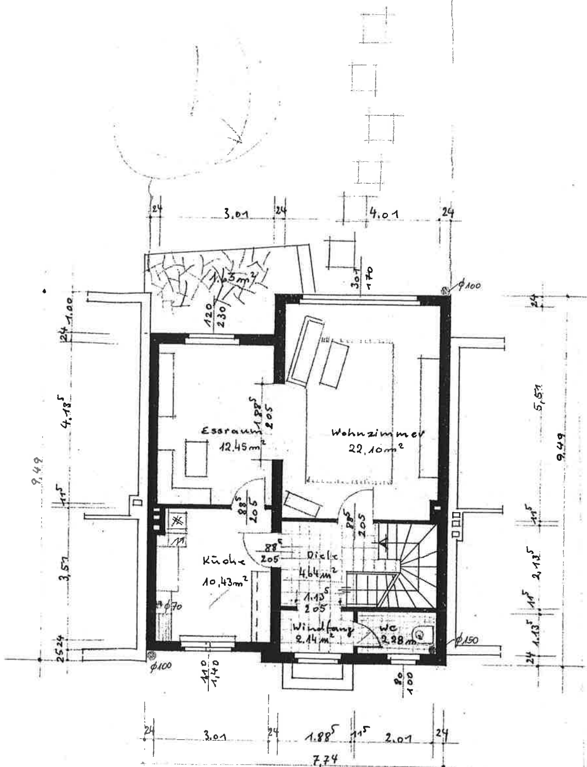
Erdgeschoß
