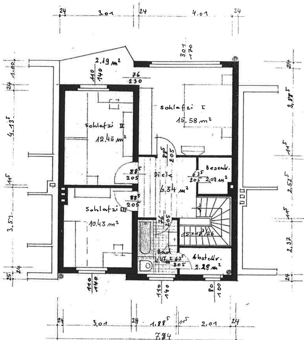
Obergeschoß
