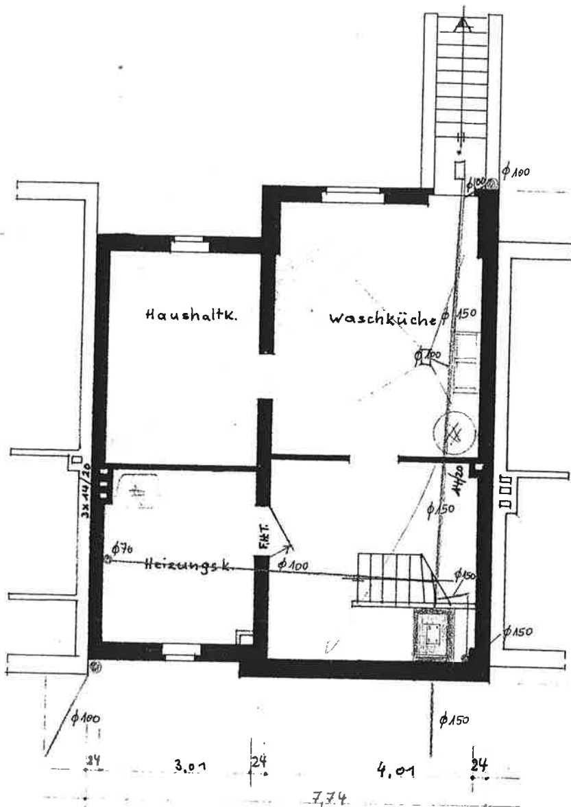
Kellergeschoß
